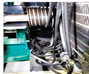
사례 2 : 팬벨트 점검 미흡으로 벨트 풀림으로 인한 파손, 탈락
